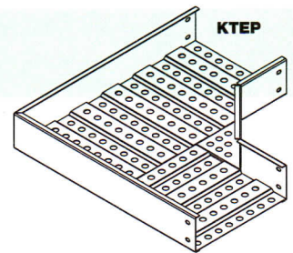
ข้องอฉาก 90° เคเบิลทรี (ข้างเดียว)
