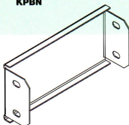
แผ่นปิดหัวท้ายเคเบิลทรี (ข้างเรียบ)
