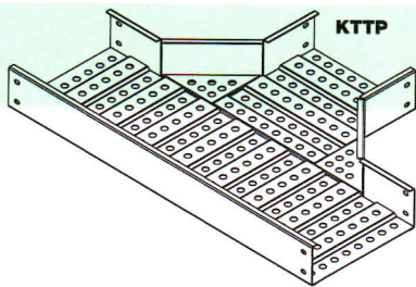
สามทางเคเบิลทรี (ข้างเรียบ)
