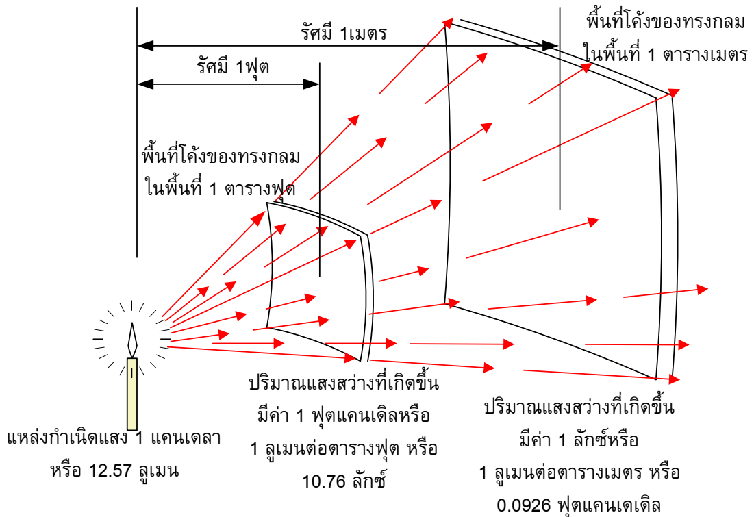
รูปที่ 2.2 แสดงปริมาณแสงที่ตกลงบนพื้นผิวทรงกลม
